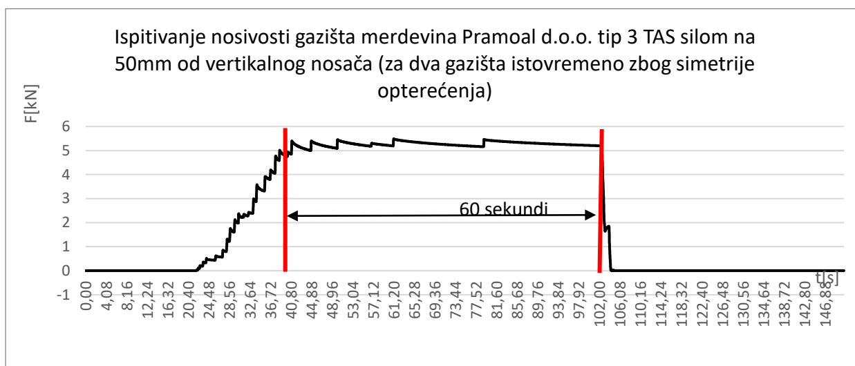
Слика 7 Запис мерног система са испитивања носивости газишта
